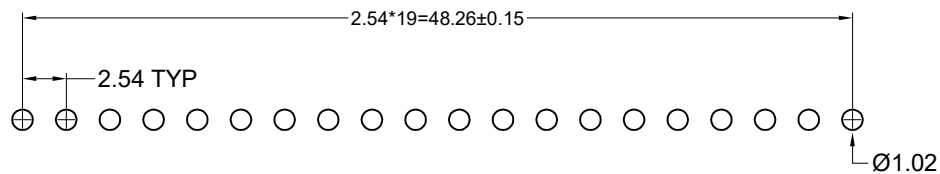
P.C.B Layout
