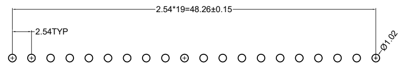
P.C.Board Layout
